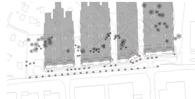
VINTERSOLSTÅND 12:00
